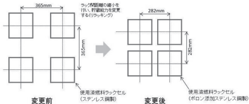
リラッキングの概念図 (原子力発電・核燃料サイクル技術等検討小委員会資料より)
